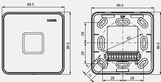
Front und Rückwand Kaba Kompaktleser 91 10
