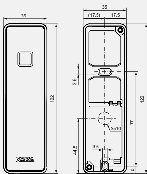
Kaba Kompaktleser 91 04, Standard-Ausführung.
