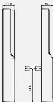
Kaba Kompaktleser 91 04, Seitenansicht; IP66-Ausführung mit Kabelabgang.
